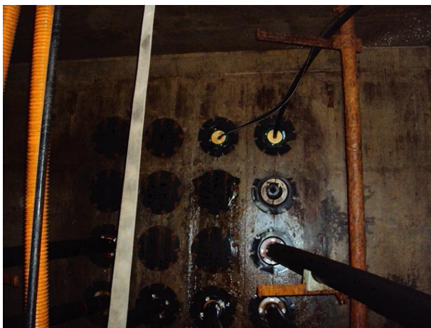
관로부 누수
