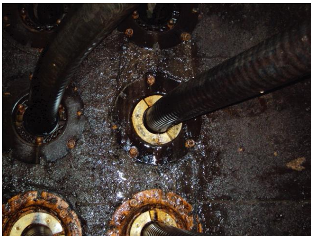
관로부 누수흔적
