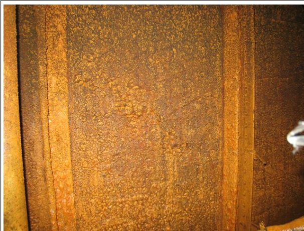
동측벽체 재료분리
