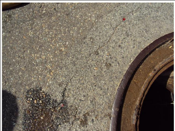
포장부 균열
