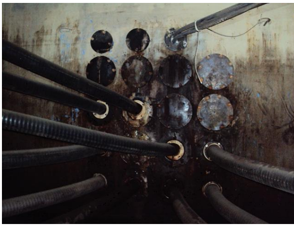
관로부 전경
