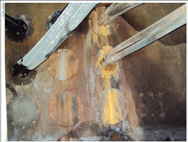
관로부 누수
