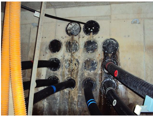
관로부 누수흔적
