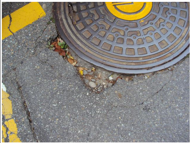
포장부 포장파손
