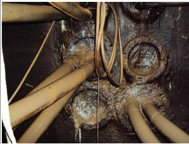
관로부 백태
