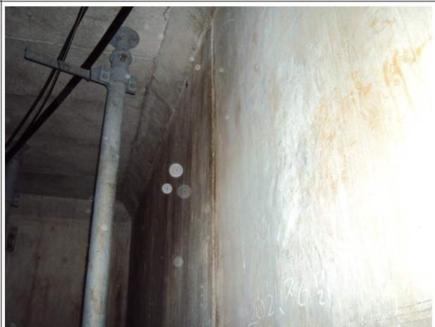
벽체 배부름
